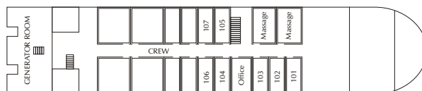
PONT INFÉRIEUR
